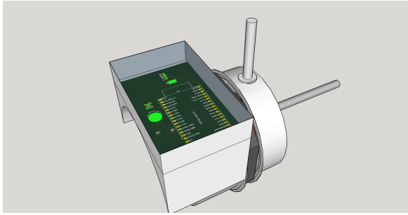
Gambar EL3.8: Lokasi instalasi sistem sensor (tampak 3/4)
