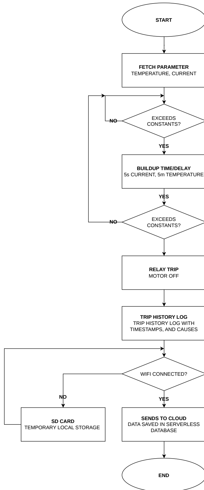
Gambar EL3.17: Flowchart Subsisitem Desain Alarm dan Sistem Proteksi
