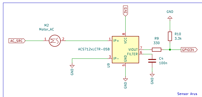
Gambar EL3.8: Skematik ACS712 ke ESP32
