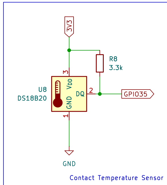
Gambar EL3.7: Skematik koneksi DS18B20 ke ESP32
