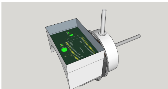
Gambar EL3.14: Lokasi instalasi sistem sensor (tampak 3/4)
