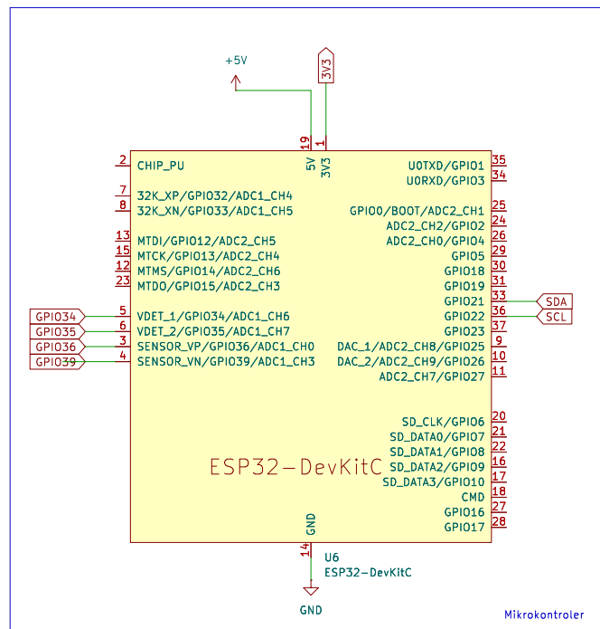
Gambar EL3.5: Skematik koneksi sistem sensor ke mikrokontroler ESP32
