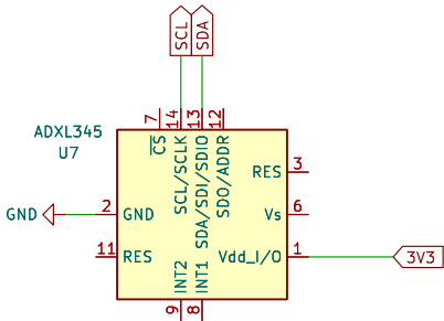
Sensor Akselerometer
