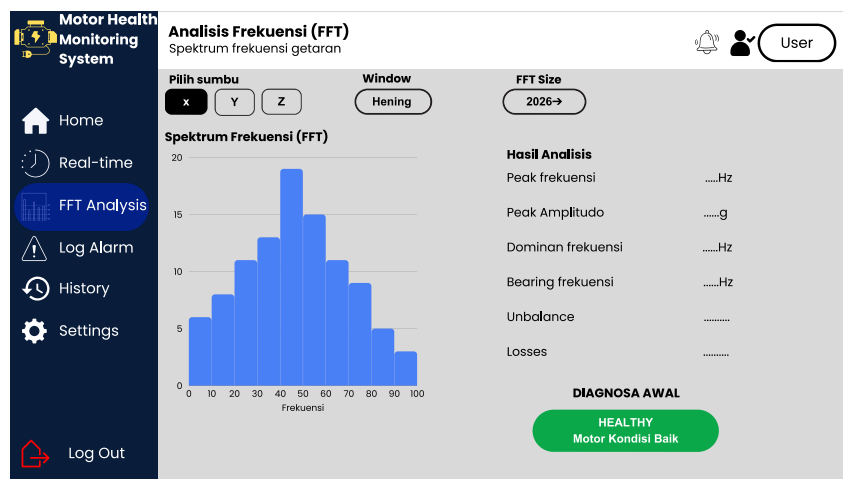
Gambar EL3.15: Laman domain frekuensi kecepatan rms
