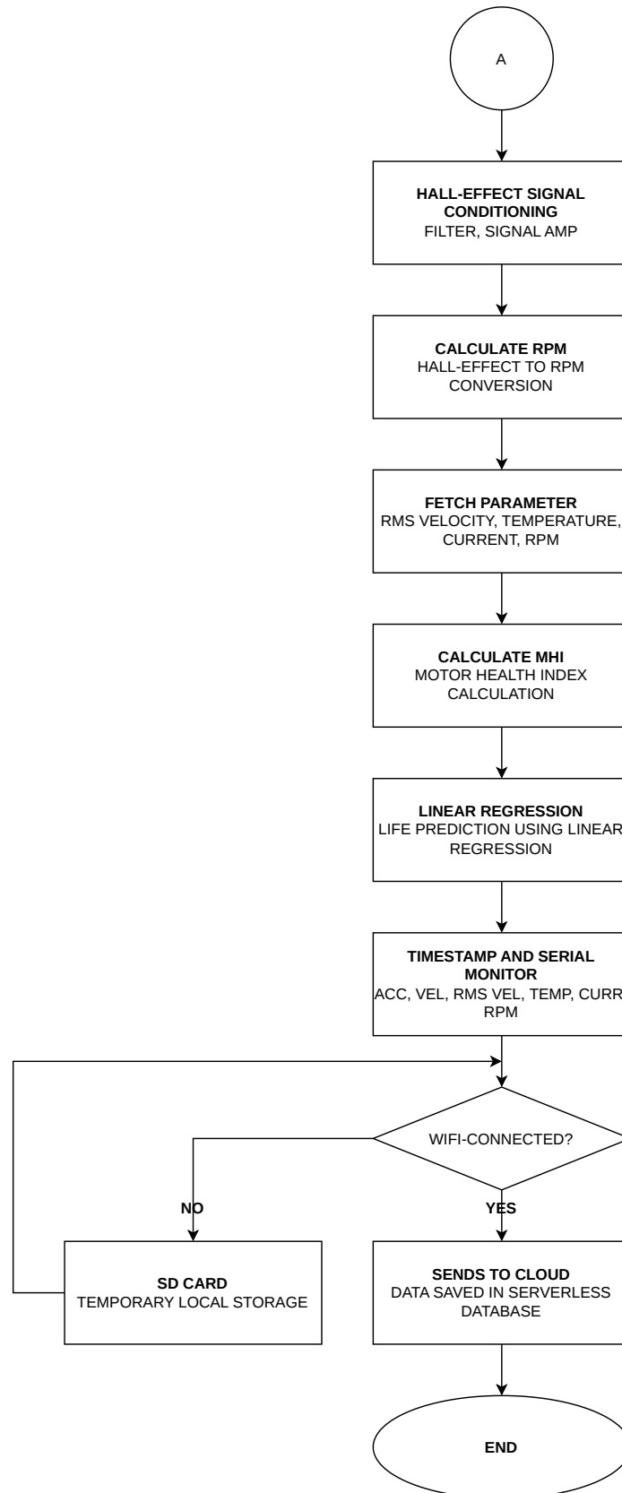
Gambar EL3.3: Flowchart Subsisitem Instalasi Sensor dan Pemrosesan Sinyal (ISPS)
