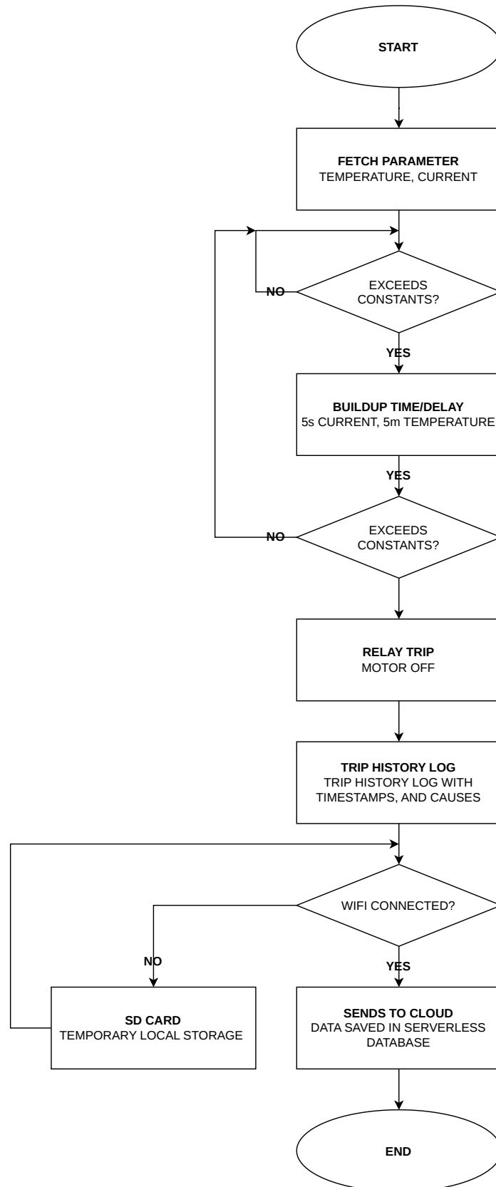
Gambar EL3.18: Flowchart Subsisitem Desain Alarm dan Sistem Proteksi
