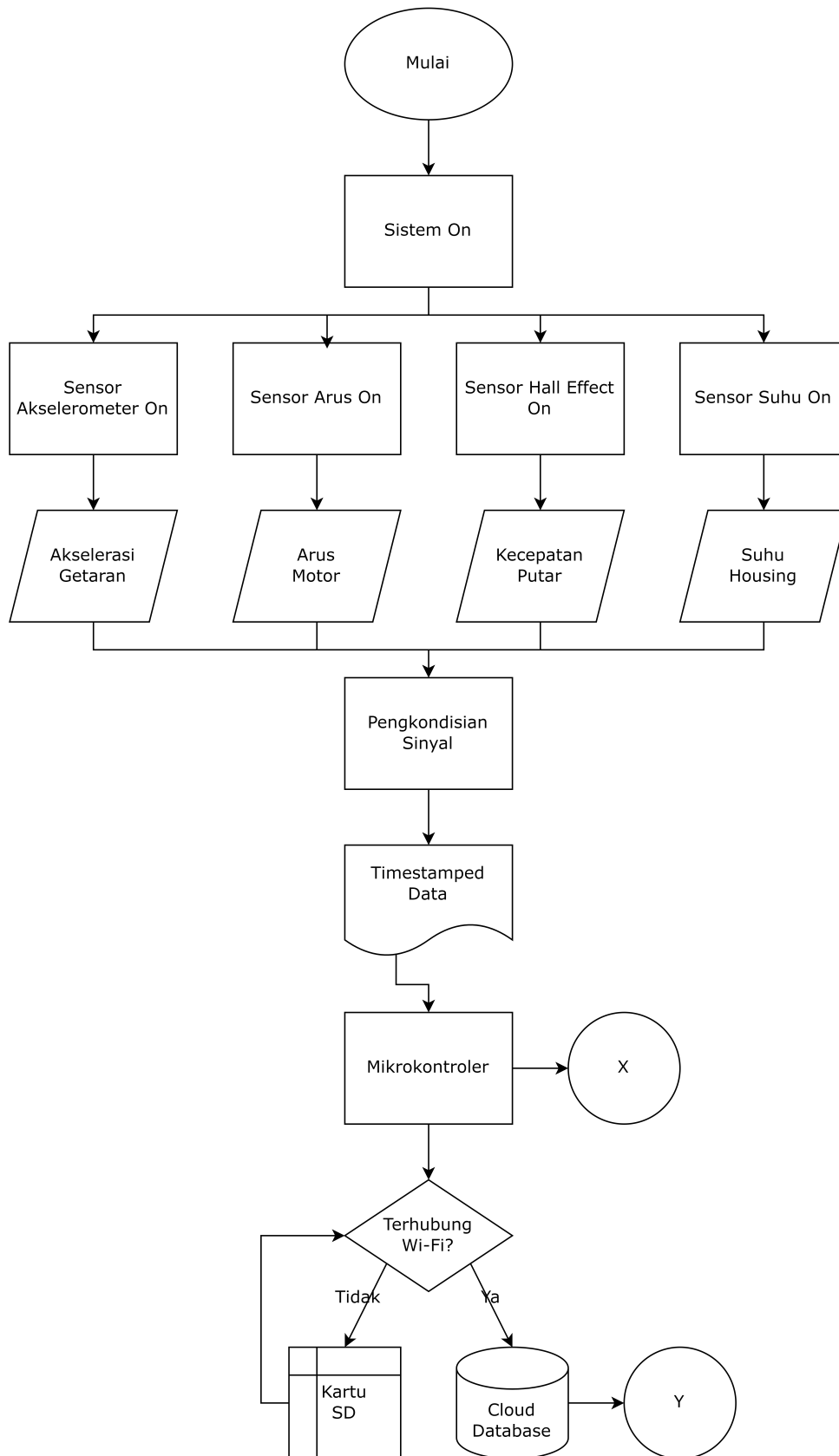
Gambar EL3.2: Flowchart Subsistem Instalasi Sensor dan Pemrosesan Sinyal (ISPS)
