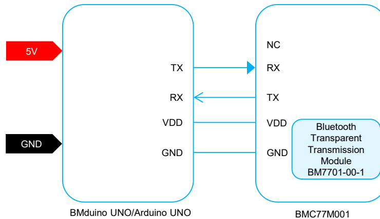
接線示意圖
