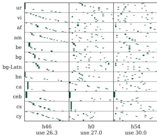
a // SONAR: ste_h76_init01, layer 0
