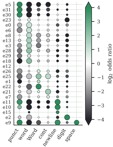
b // GPT-2 layer 0, head 15
