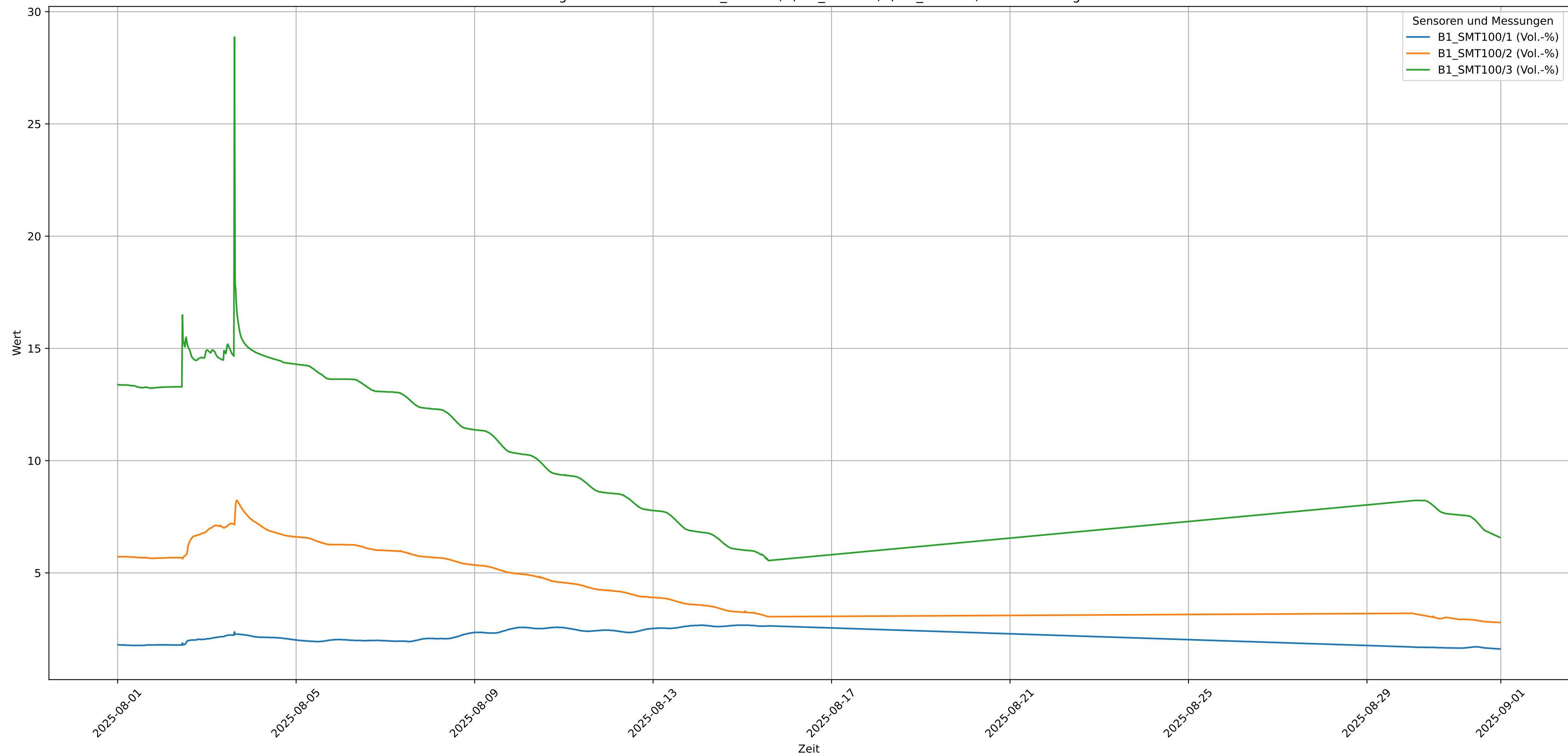
Zeit-Wert-Diagramm für Sensoren: B1_SMT100/1, B1_SMT100/2, B1_SMT100/3 und Messungen: Vol.-%
