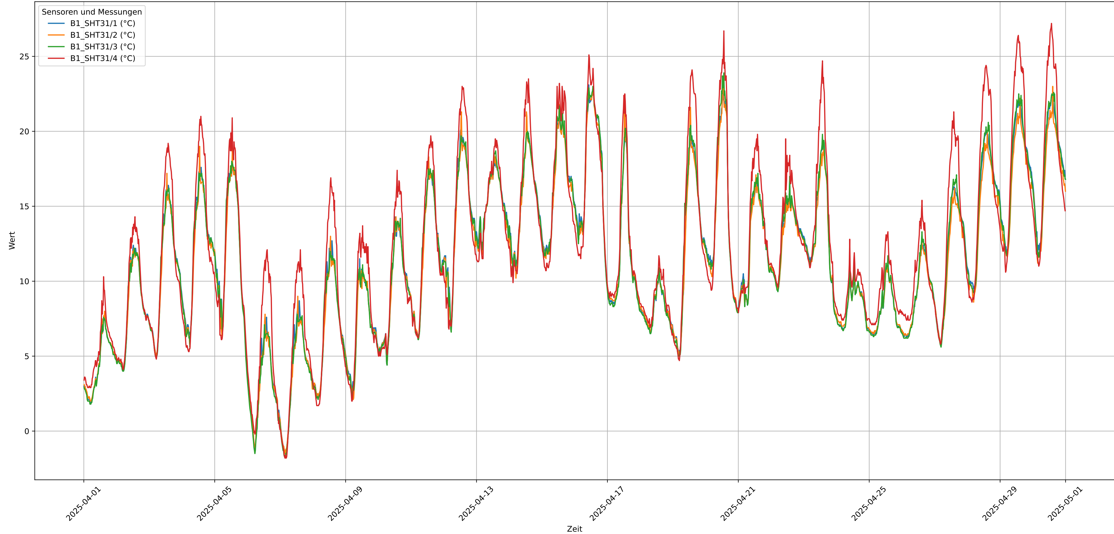
Zeit-Wert-Diagramm für Sensoren: B1_SHT31/1, B1_SHT31/2, B1_SHT31/3, B1_SHT31/4 und Messungen: °C
