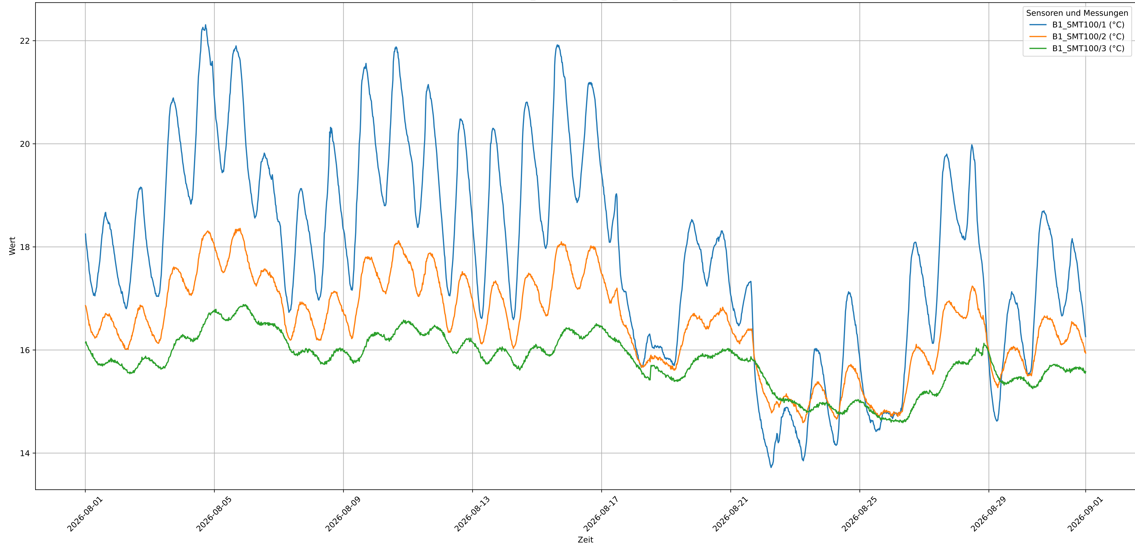
Zeit-Wert-Diagramm für Sensoren: B1_SMT100/1, B1_SMT100/2, B1_SMT100/3 und Messungen: °C
