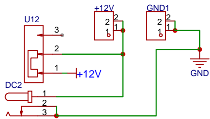
电源接口
