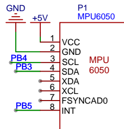
陀螺仪模块
