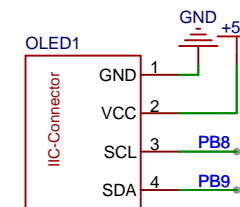
OLED屏幕
