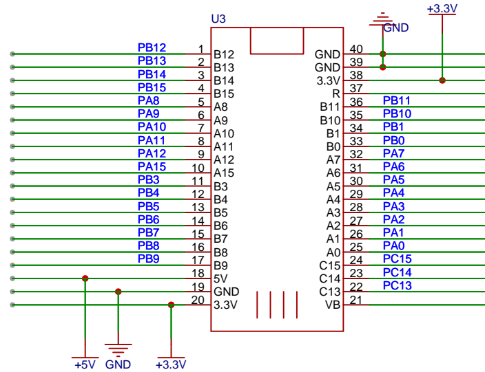
单片机
