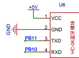
蓝牙模块
