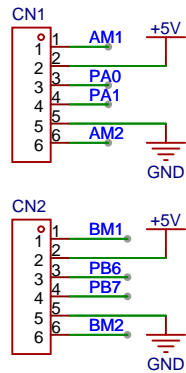
电机接口
