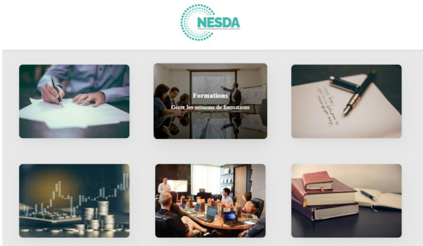
Figure 3.2 page d'accueil
