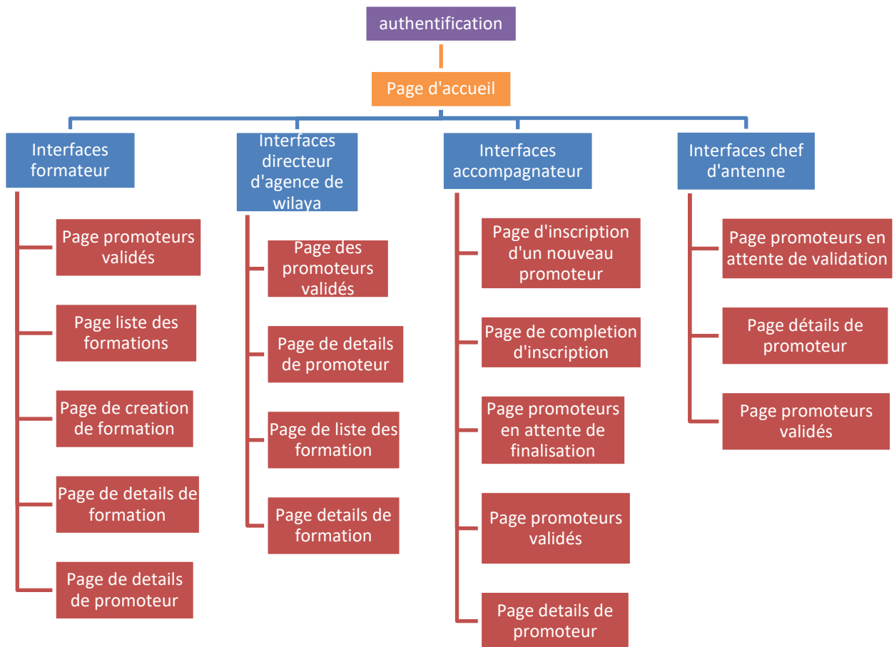
Figure 2.1 schéma d'arborescence
