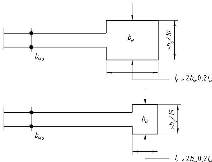
Figure 5.10 — Épaisseur minimale des éléments de rive confinés
