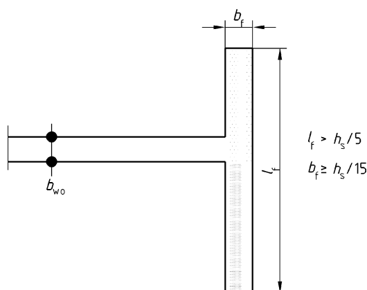
Figure 5.9 — Élément de rive confiné inutile à une extrémité du mur avec membrure transversale importante
