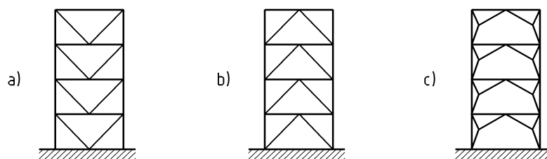
Figure 6.3 — Ossatures avec entretoises centrées en V (zones dissipatives dans les diagonales tendues et comprimées)
