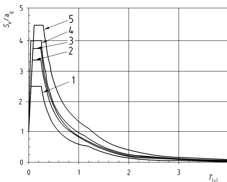
Figure 3.3 — Spectres de réponse élastique de type 2 recommandés pour les sols de classes A à E (à 5 % d'amortissement)
