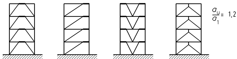
Figure 6.4 — Ossatures avec entretoises excentrées (zones dissipatives dans les tronçons d'excentrement fléchis ou cisailés). Valeurs par défaut pour a_u/a_1 (voir 6.3.2(3) et Tableau 6.2)
