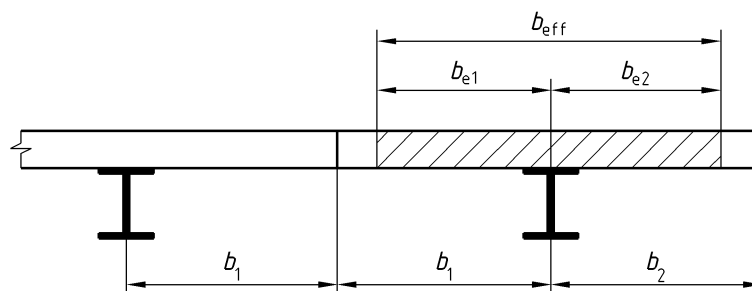
Figure 7.6 — Définition des largeurs participantes b_e et b_{eff}
