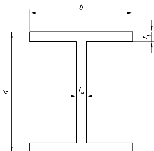
Figure 6.13 — Définitions des notations pour les sections de tronçons en I
