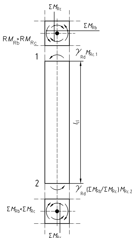
Figure 5.2 — Valeurs dues au dimensionnement en capacité pour l'effort tranchant dans les poteaux
