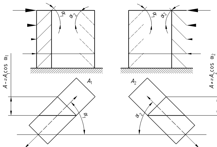
Figure 6.12 — Exemple d'application de 6.7.1(3)
