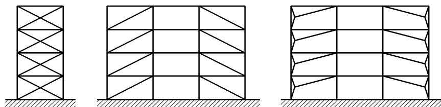
Figure 6.2 — Ossatures avec entretoises diagonales centrées (zones dissipatives dans les diagonales tendues uniquement)
