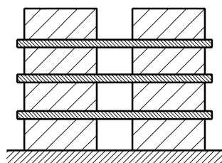
Figure 7.2 — Systèmes structuraux mixtes. Type 3 — murs mixtes ou en béton couplés à des poutres en acier ou mixtes
