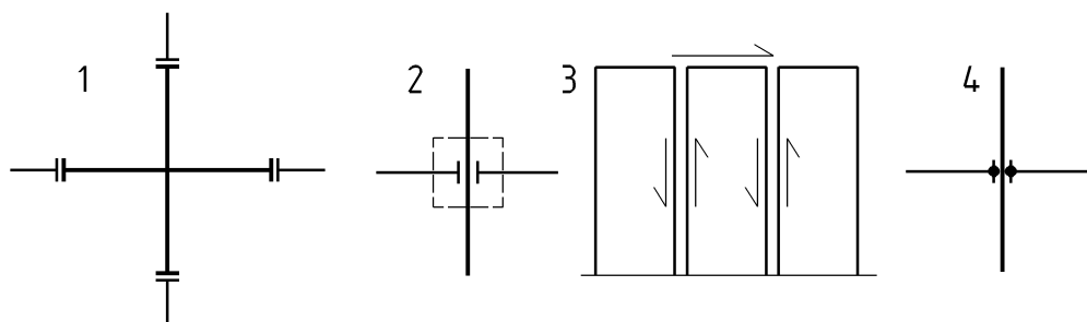
Figure 5.14 — a) assemblages situés en dehors des zones critiques, b) assemblages surdimensionnés, les rotules plastiques étant situées hors des assemblages, c) assemblages ductiles à l'effort tranchant, entre panneaux de grandes dimensions, situés à l'intérieur des zones critiques (par exemple au rez-de-chaussée) et d) assemblages ductiles de continuité situés à l'intérieur des zones critiques des ossatures
