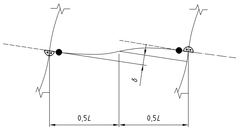
Figure 6.11 — Flèche de la poutre pour le calcul de \theta_p
