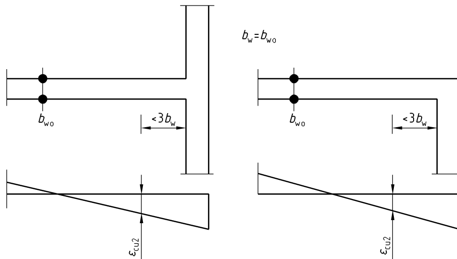
Figure 5.11 — Épaisseur minimale des éléments de rive confinés dans les murs de DCH avec de larges ailes
