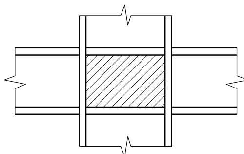
Figure 6.10 — Panneau d'âme encadré par des semelles et des raidisseurs
