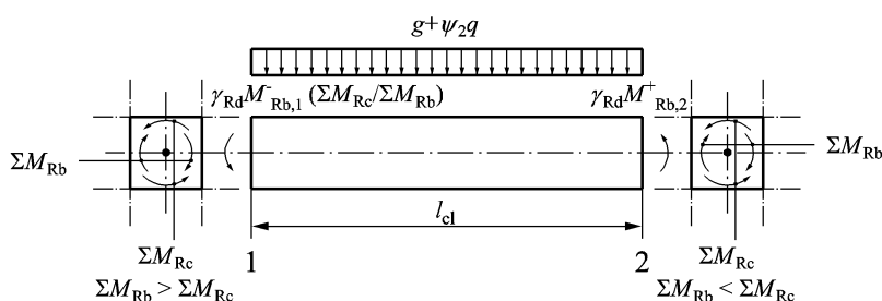
Figure 5.1 — Valeurs dues au dimensionnement en capacité pour l'effort tranchant dans les poutres
