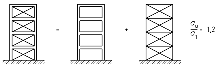
Figure 6.7 — Ossature en portique combinée avec une triangulation centrée (zones dissipatives dans l'ossature en portique et dans les diagonales tendues). Valeurs par défaut pour a_u/a_1 (voir 6.3.2(3) et Tableau 6.2)
