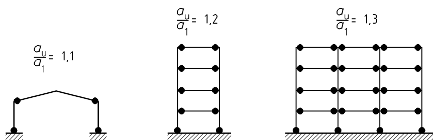
Figure 6.1 — Ossatures en portique (zones dissipatives dans les poutres et en pied de poteaux). Valeurs par défaut pour \alpha_u/\alpha_1 (voir 6.3.2(3) et Tableau 6.2)
