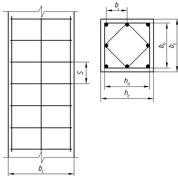
Figure 5.7 — Confinement du noyau de béton
