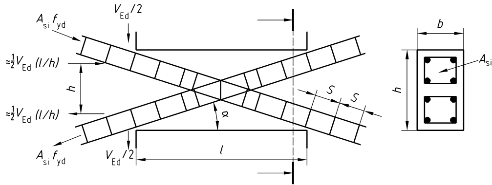
Figure 5.12 — Linteau avec armatures diagonales
