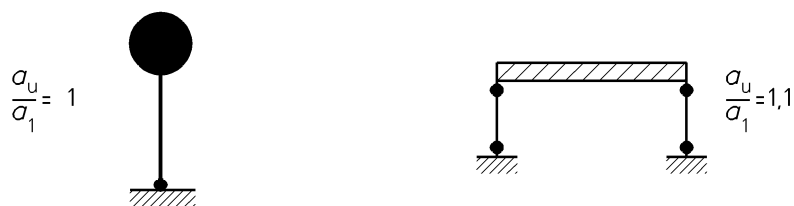
Figure 6.5 — Pendule inversé : a) zones dissipatives à la base des poteaux ; b) zones dissipatives dans les poteaux ( N_{Ed}/N_{pl,Rd} < 0,3 ). Valeurs par défaut pour a_u/a_1 (voir 6.3.2(3) et Tableau 6.2)
