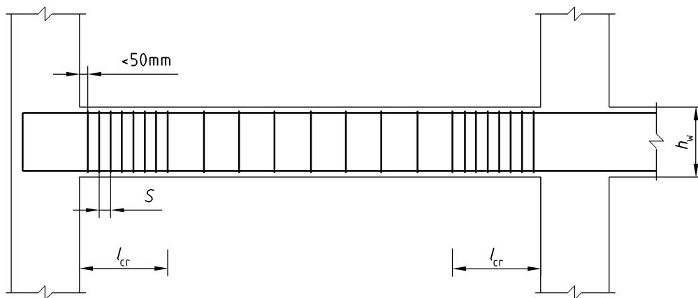
Figure 5.6 — Armatures transversales dans les zones critiques des poutres
