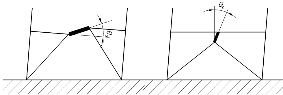
Figure 6.14 — a) moments égaux aux extrémités du tronçon ; b) moments inégaux aux extrémités du tronçon
