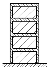
Figure 6.8 — Ossature en portique combinée avec des remplissages
