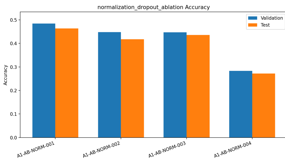
图 4: 归一化与 Dropout 消融准确率对比
