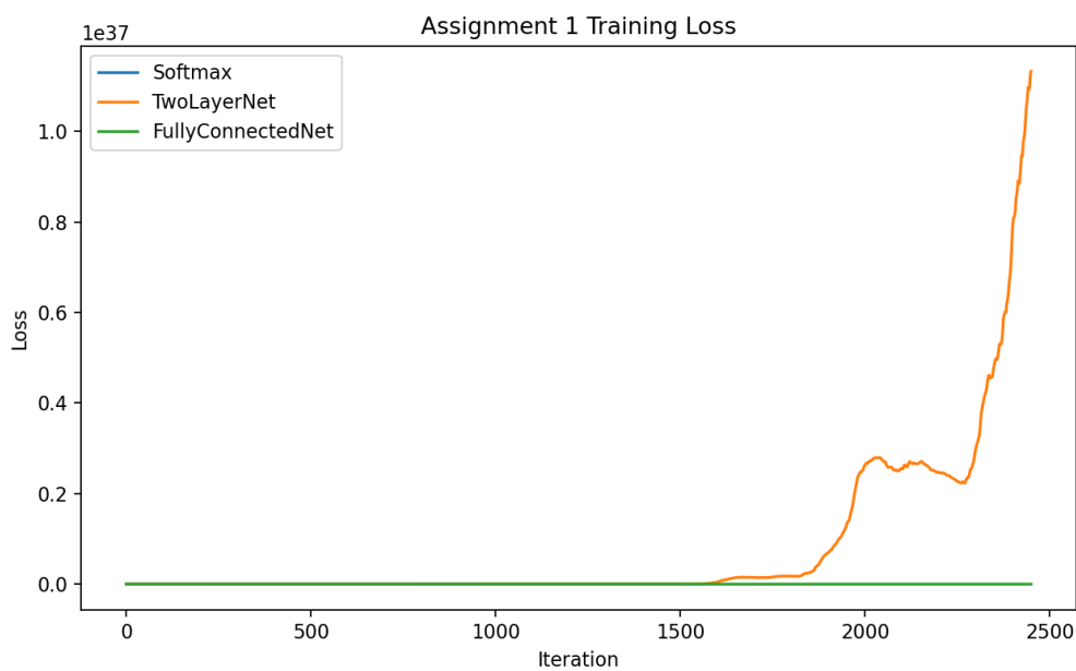
图 1: Assignment 1 baseline 训练损失曲线
