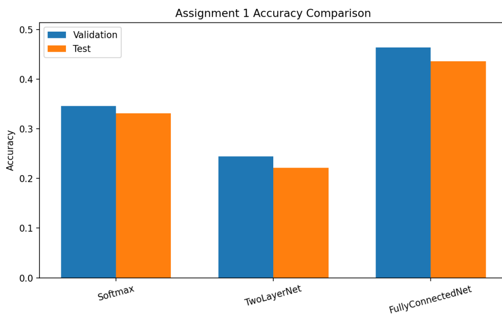
图 2: Assignment 1 baseline 验证集与测试集准确率对比
