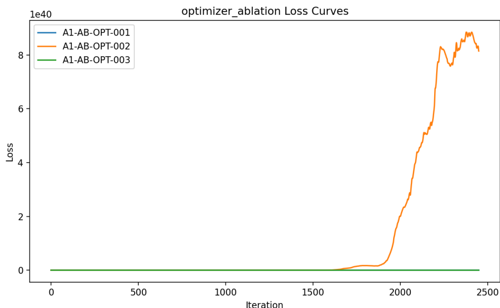
图 3: 优化器消融损失曲线
