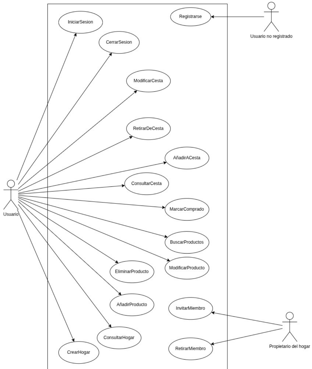
Figura 4. Diagrama general de casos de uso
