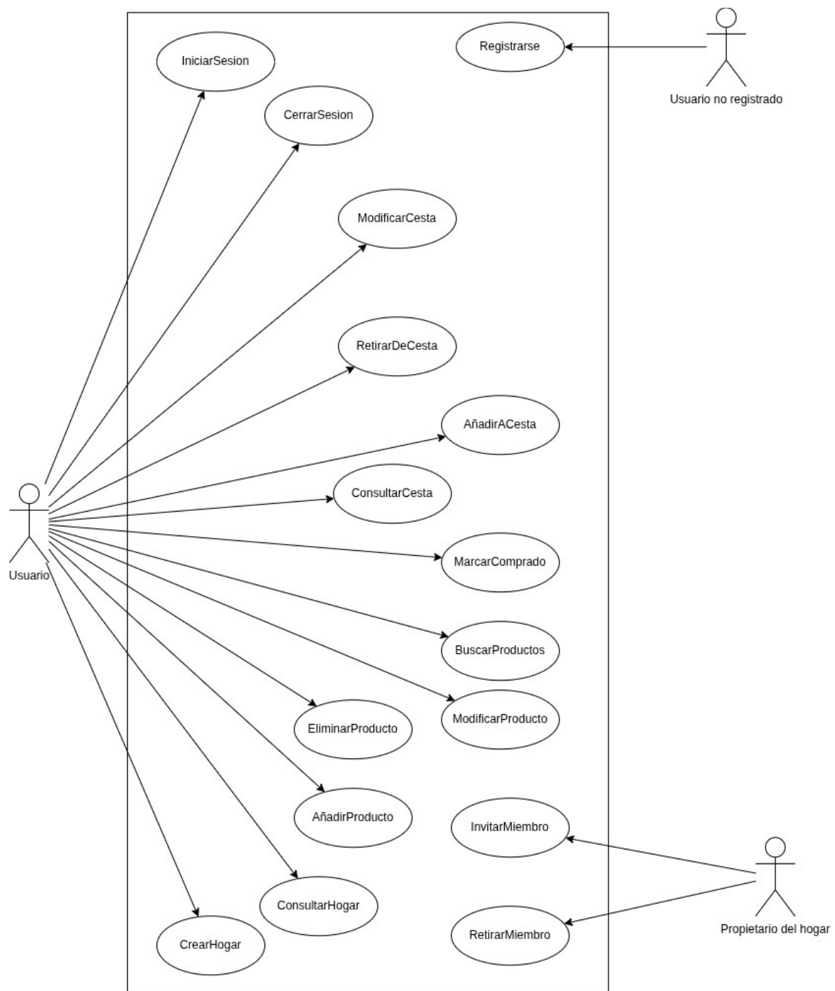
Anexo I — Figura A1. Diagrama general de casos de uso
