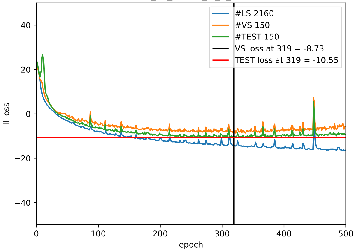
II_pv_UMNN_M_3_0
