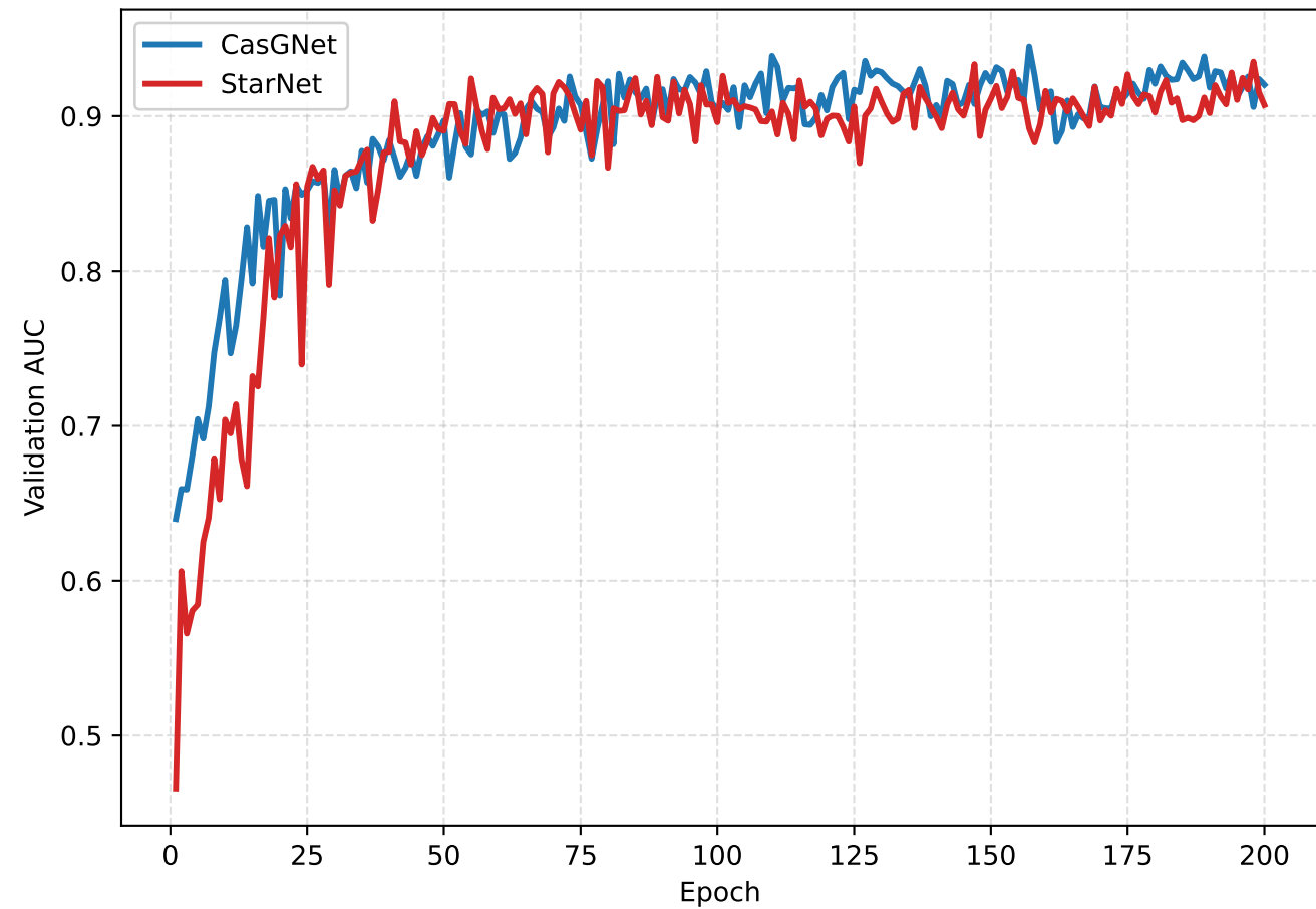
Validation AUC
