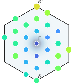
b n_1(\mathbf{k})
