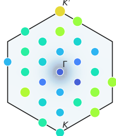
f n_1(\mathbf{k})
