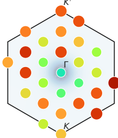
j n_1(\mathbf{k})
