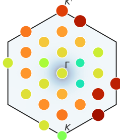
n n_1(\mathbf{k})
