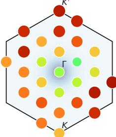
j n_1(\mathbf{k})
