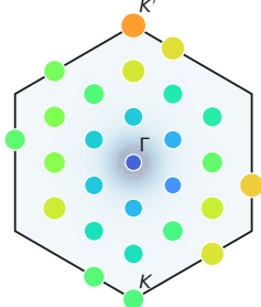
e n_{\text{tot}}(\mathbf{k}) : 8.85 \pm 0.082
