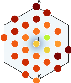
m n_{\text{tot}}(\mathbf{k}) : 18.0 \pm 0.19
