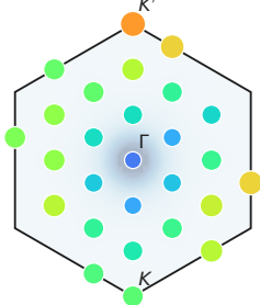
a n_{\text{tot}}(\mathbf{k}) : 8.91 \pm 0.080
