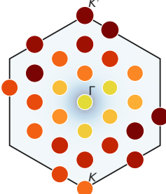
i n_{\text{tot}}(\mathbf{k}) : 17.9 \pm 0.2
