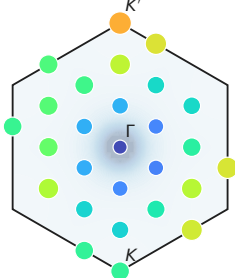
f n_1(\mathbf{k})
