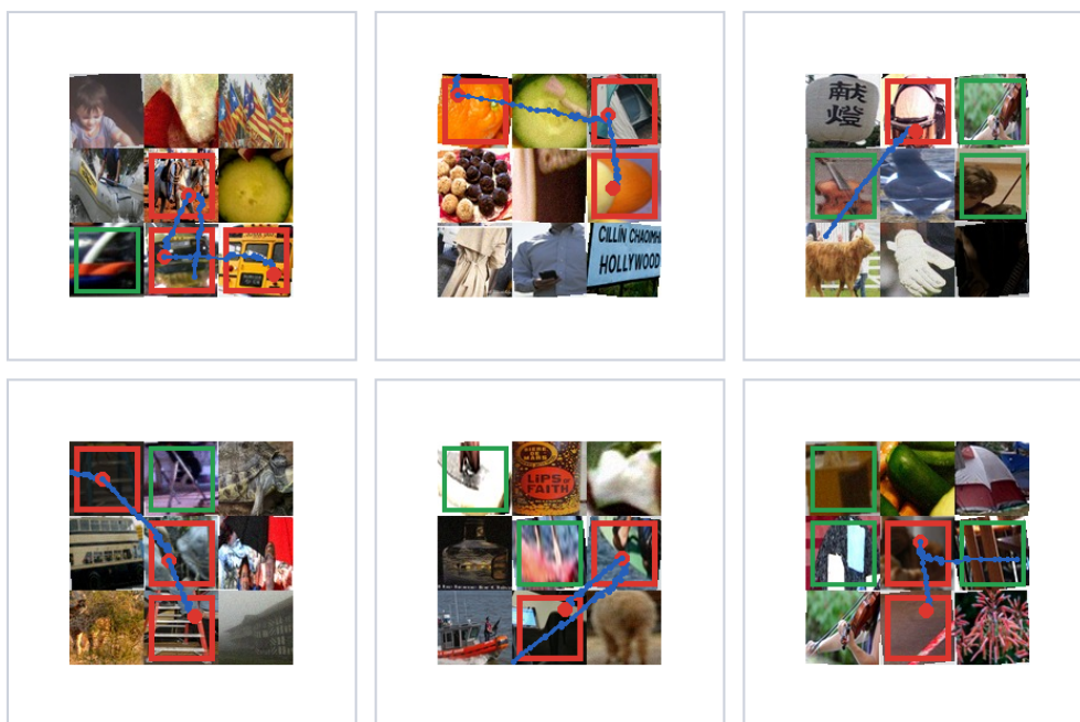
图 10: Qwen3-VL-Flash baseline 的失败样例拼图。通用 VLM 能识别部分目标，但在低分辨率九宫格、严格格子编号和多目标集合输出上容易出现漏点或多点。
