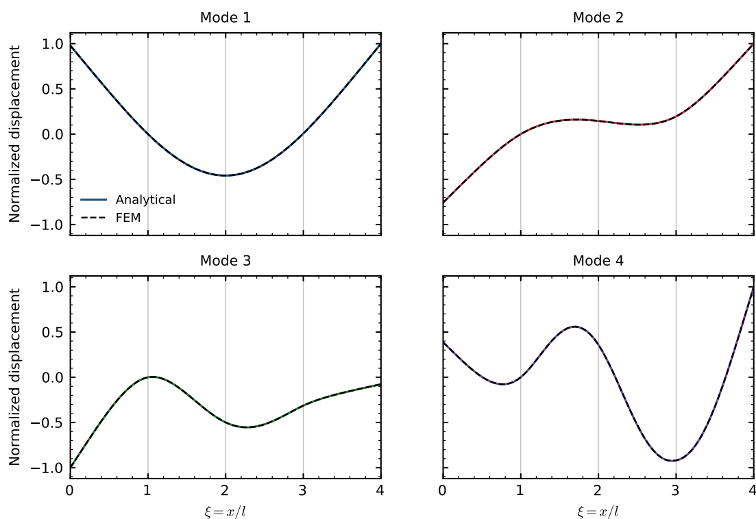
图 3: 前四阶振型叠合对比
