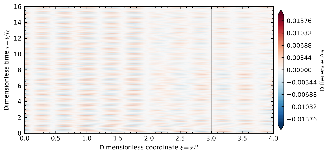
图 7: 全梁时空响应差值云图
