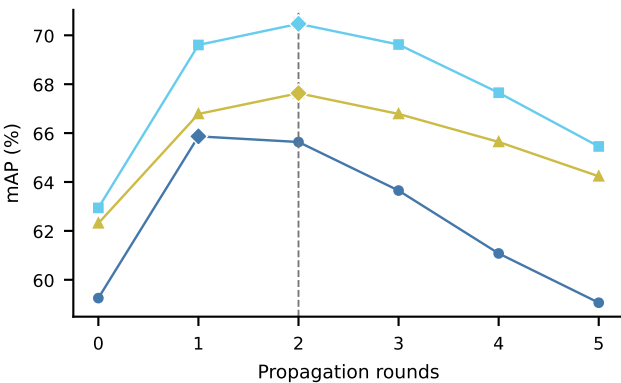
OS-ABO-core
