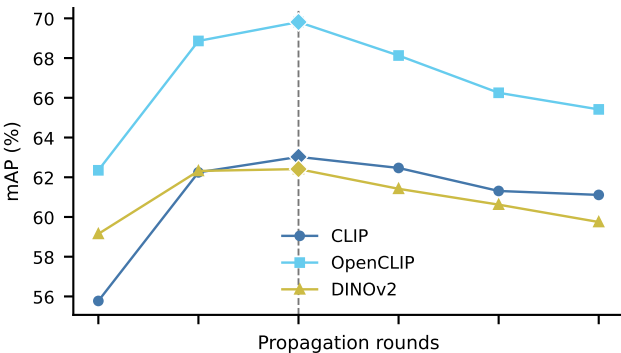
OS-ABO-core
