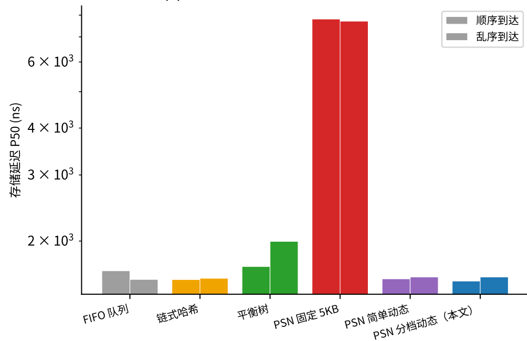
(c) 存储延迟 ( L=1024 , 固定 5KB 慢 5\times )
