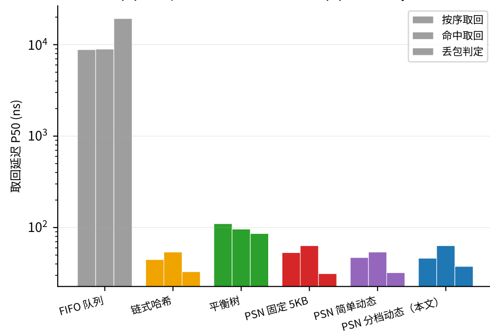
(d) 取回/丢包判定延迟 (FIFO O(n) 重排 8.8\mu s )
