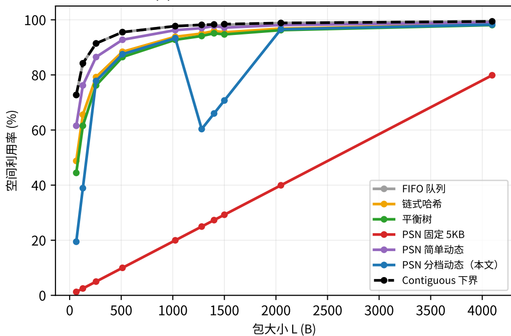
(a) 空间利用率 vs 包大小 (固定 5KB 贴地)
