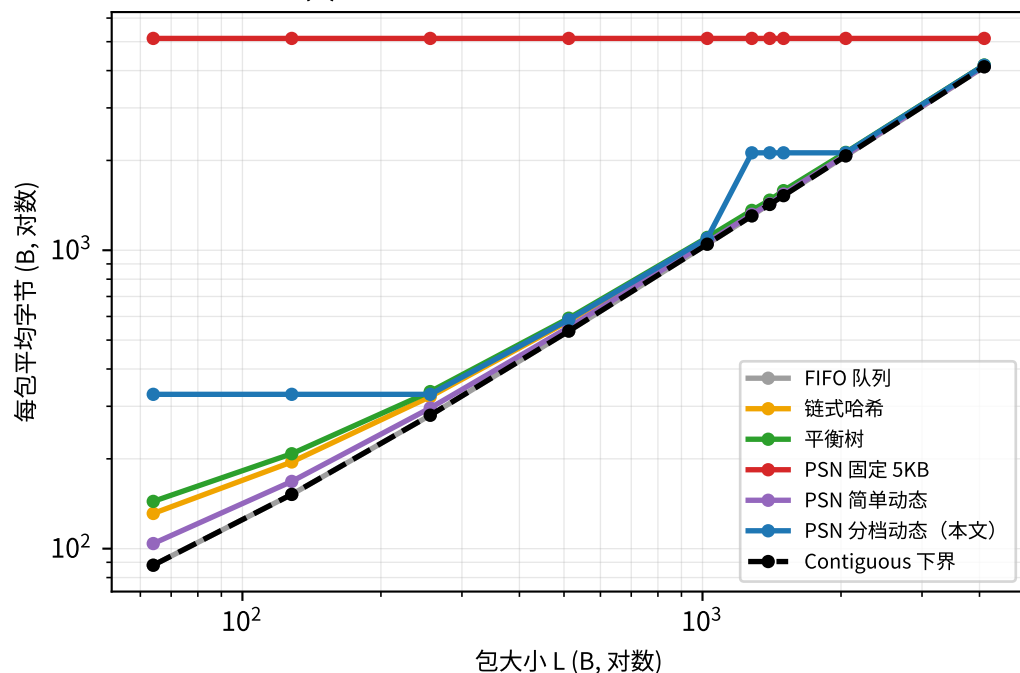
(b) 每包平均分配字节 (固定 5KB 绝对浪费)
