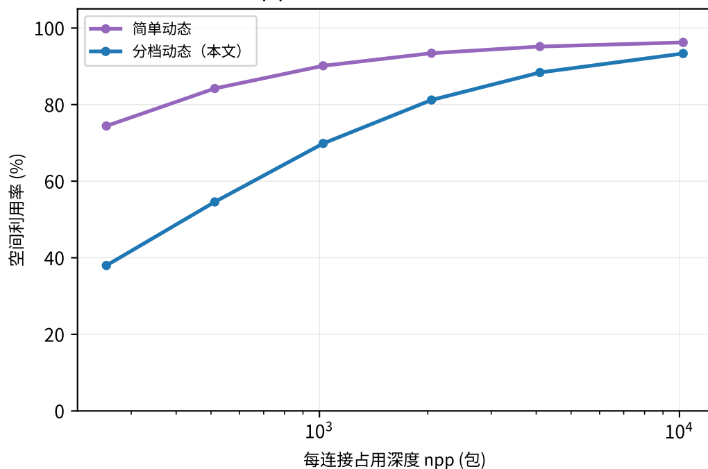
(d) 固定数组开销随占用深度摊销
