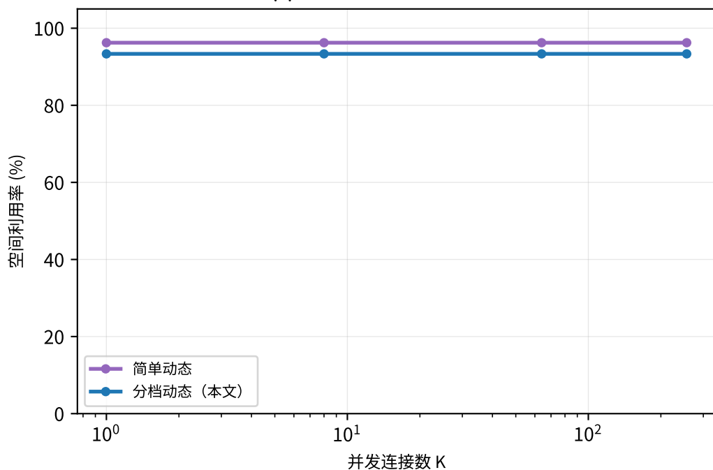
(c) 多流：利用率与连接数无关
