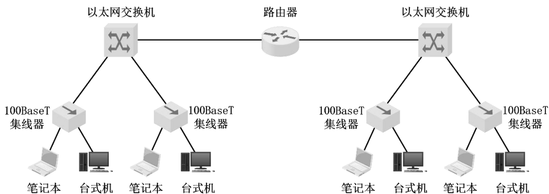
图 4-156 习题 4-107 的图
