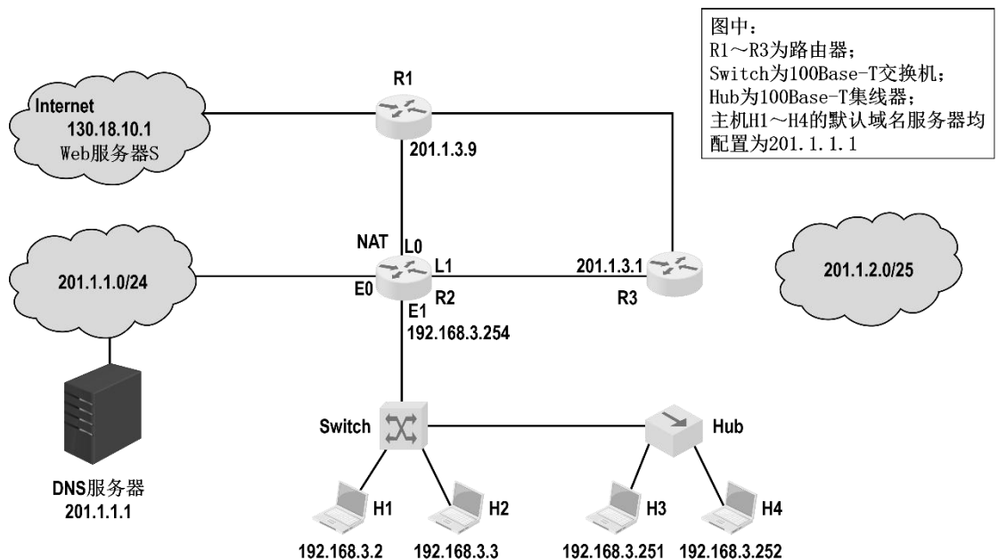
图 4-155 习题 4-97、4-98、4-99、4-100 的图
