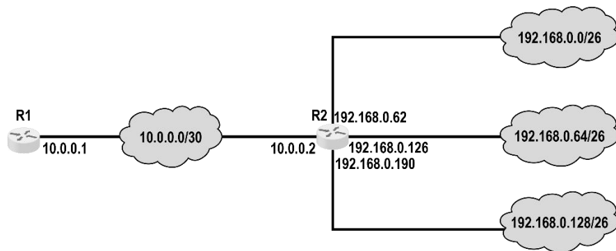
图 4-147 习题 4-57 的图
