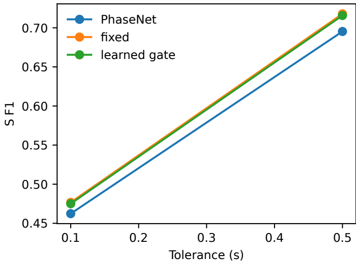
Stage 3: S F1 vs tolerance
