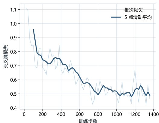
(a) 训练损失变化
