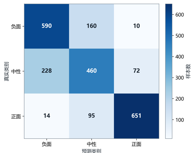
图 4 multilingual BERT 独立测试集混淆矩阵
