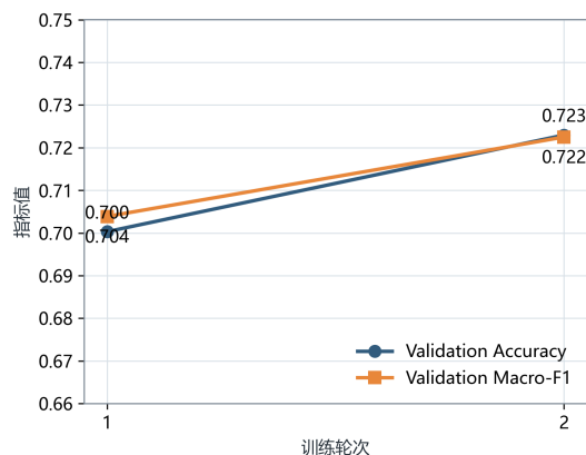
(b) 验证集 Accuracy 与 Macro-F1 变化
