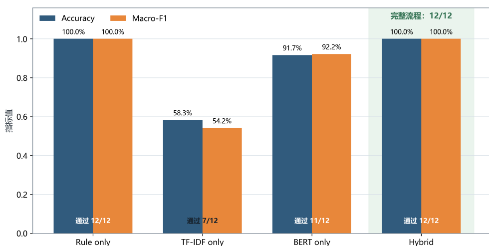
图 6 固定案例演示集消融结果：用于流程验证，不作为泛化能力指标
