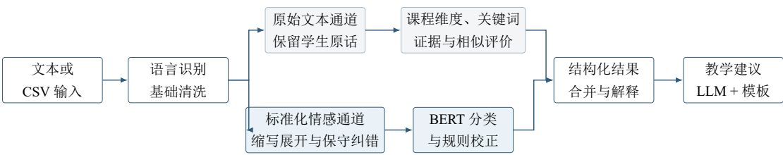
图 2 CourseInsight 双文本通道与核心数据流
