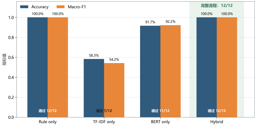
图 6 固定案例演示集消融结果
