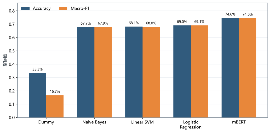
图 3 独立测试集情感分类模型对比
