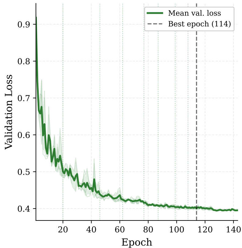
GRU
