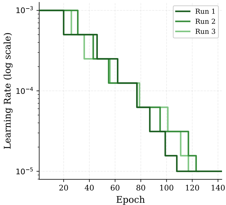
GRU
