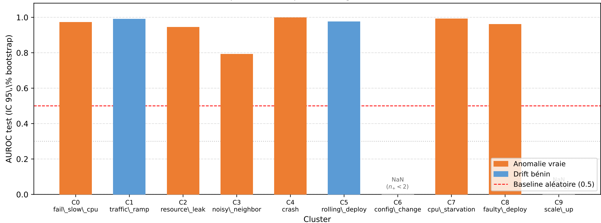
AUROC précurseur H3 par cluster (graine 42, k^* sur val)
