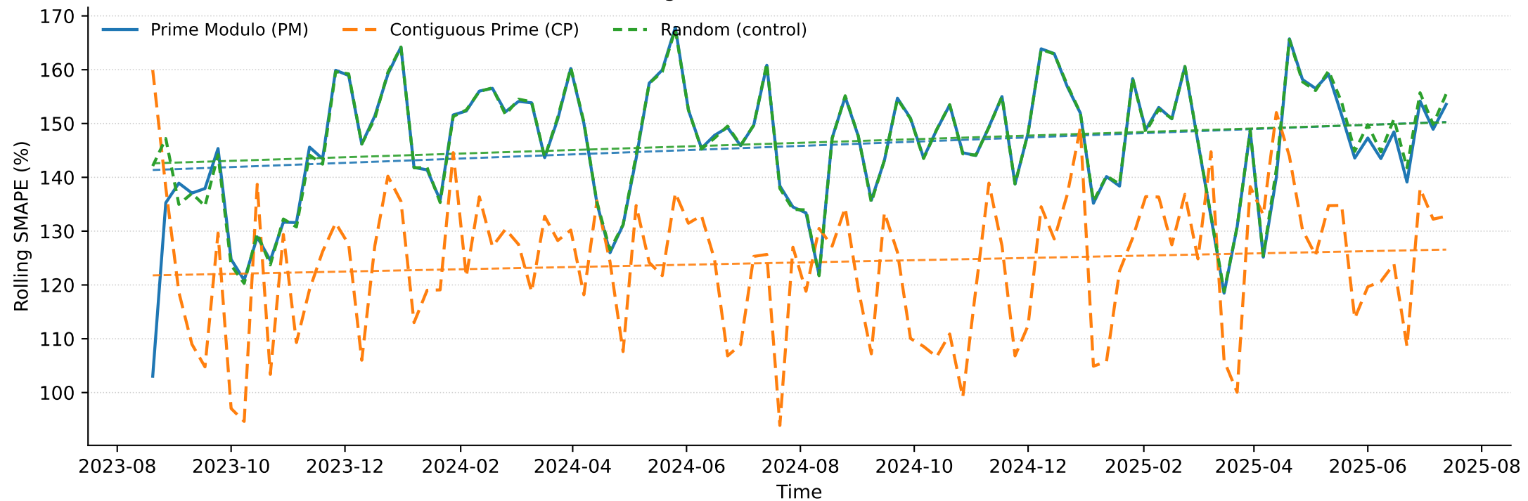
Rolling SMAPE (window=78) — SPY
