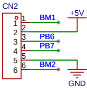
电机接口
