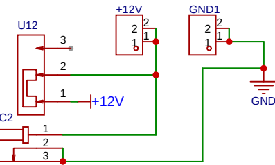
电源接口
