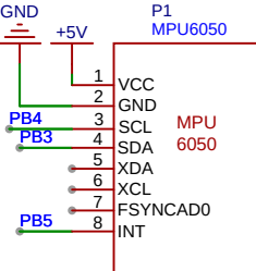
陀螺仪模块
