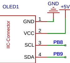
OLED屏幕
