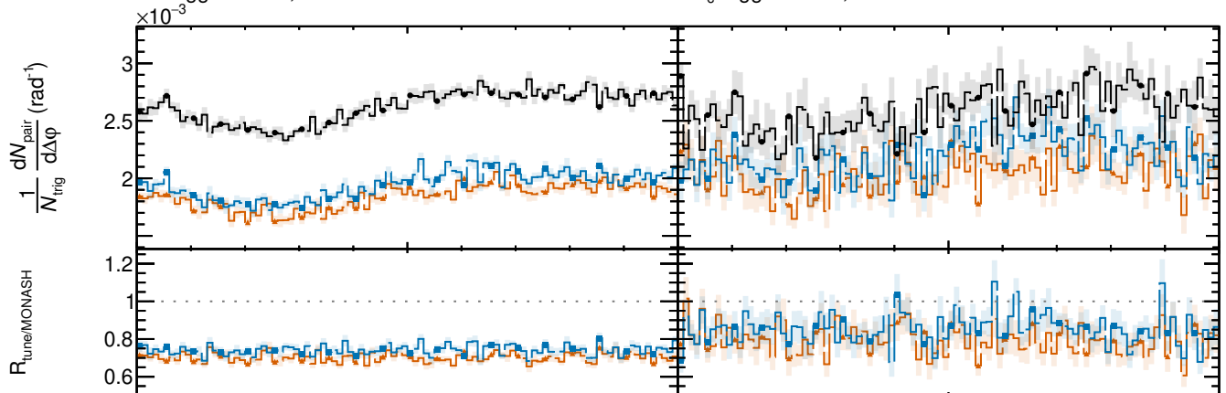
D^0 trigger \rightarrow D^0 , SS
