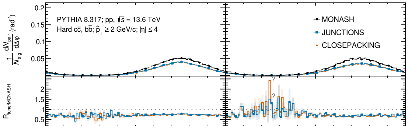
(a) B^+ trigger \rightarrow B^- , OS
