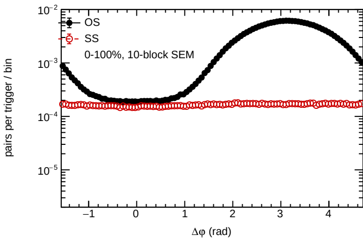
D^+ trigger
