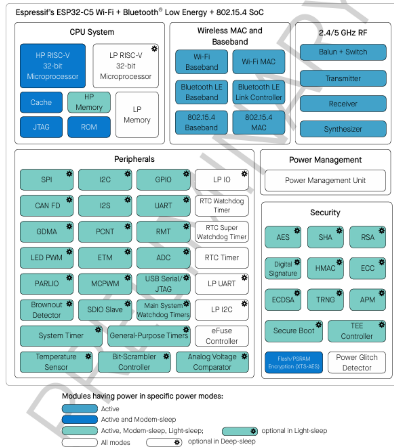
ESP32-C5 功能框图
