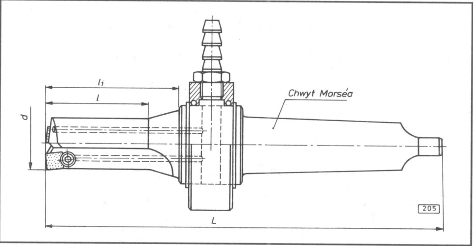
C – wiertła z doprowadzeniem chłodziwa z pierścieniem obrotowym
