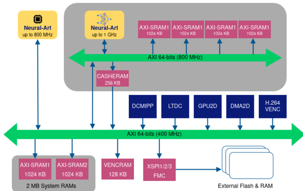
Abbildung 2.1.: STM32N6570-DK - Architektur — [10]
