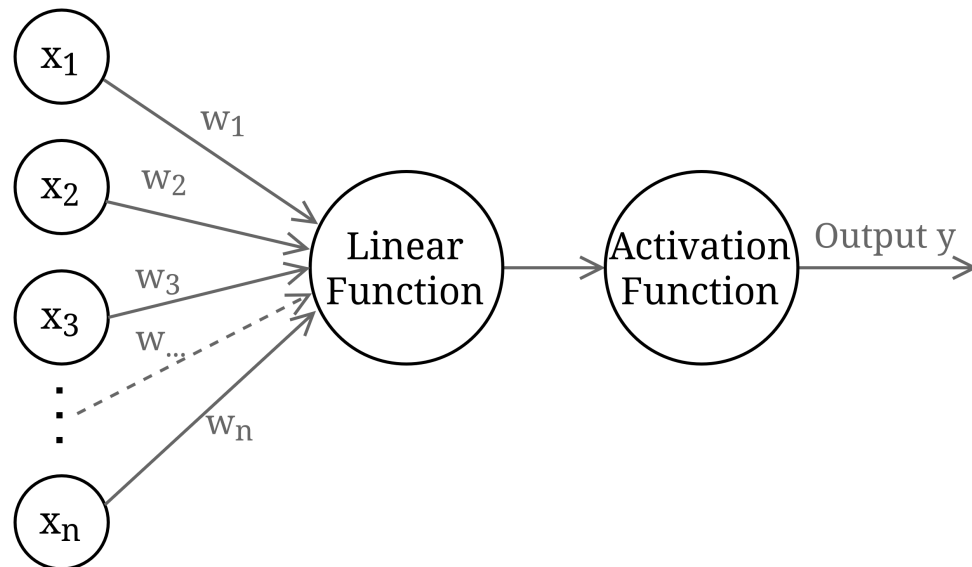
Abbildung 2.3.: Mathematisch modelliertes Neuron ([26]) — Eigene Darstellung
