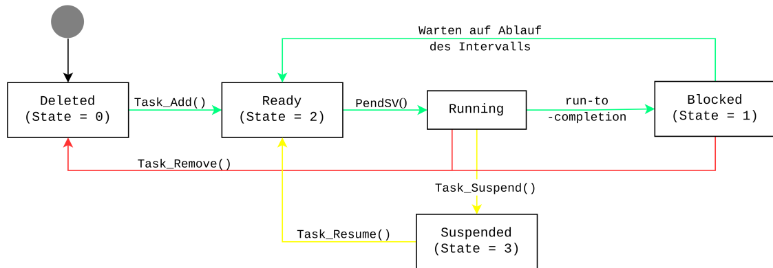
Abbildung 7.4.: Task-States des Schedulers
