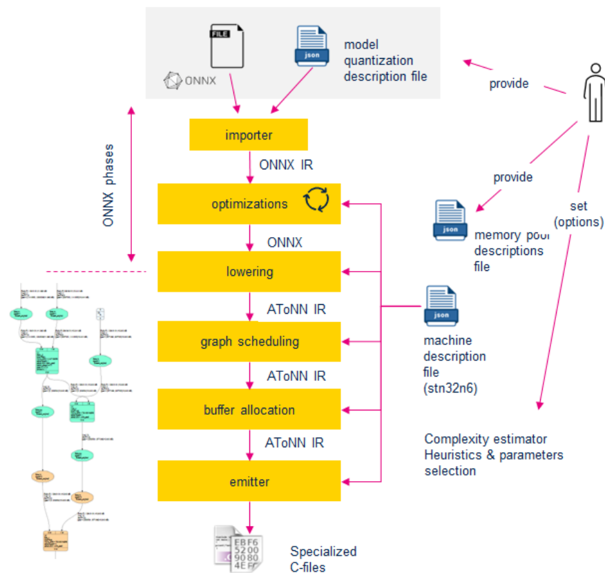
Abbildung 2.8.: NPU – Compilation [32]
