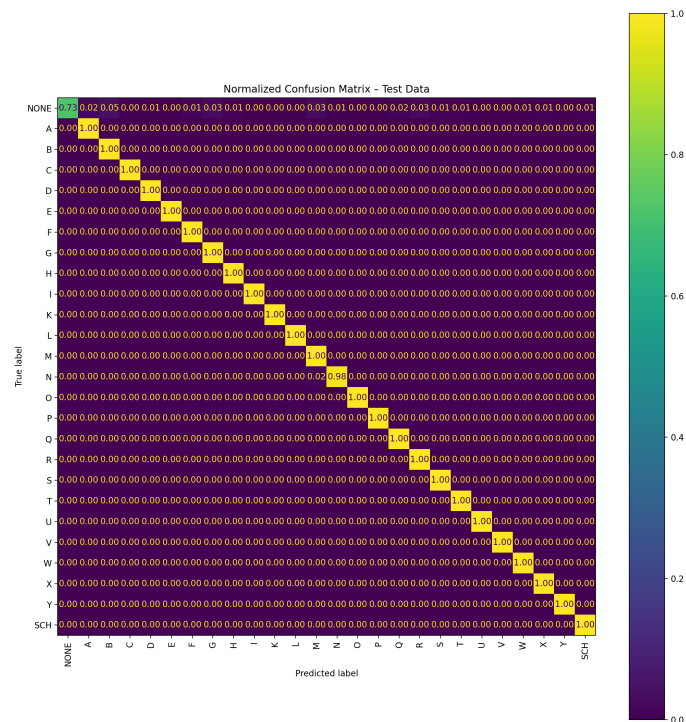
Abbildung 8.2.: Normalisierte Konfusionsmatrix
