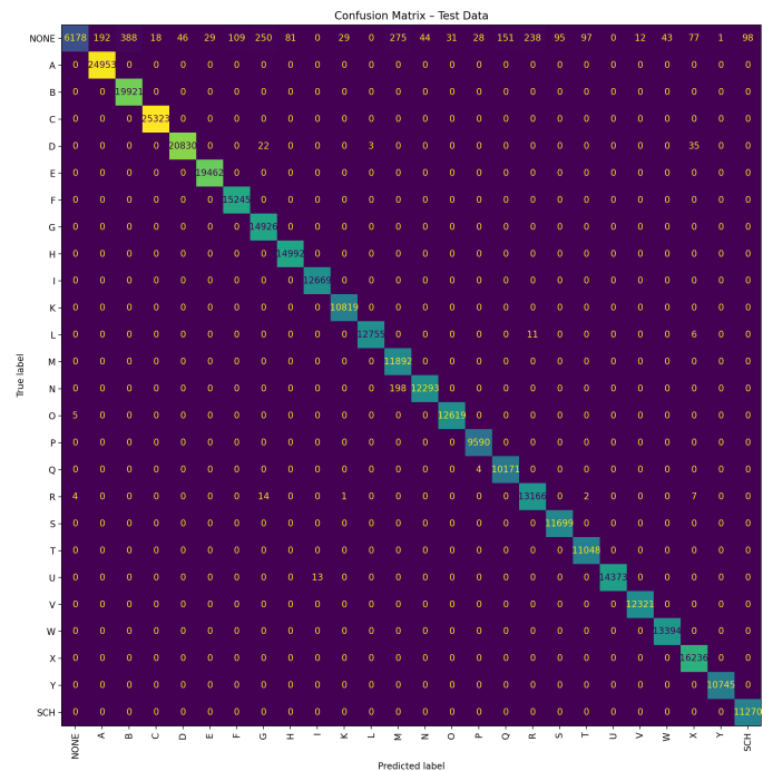
Abbildung 8.1.: Konfusionsmatrix
