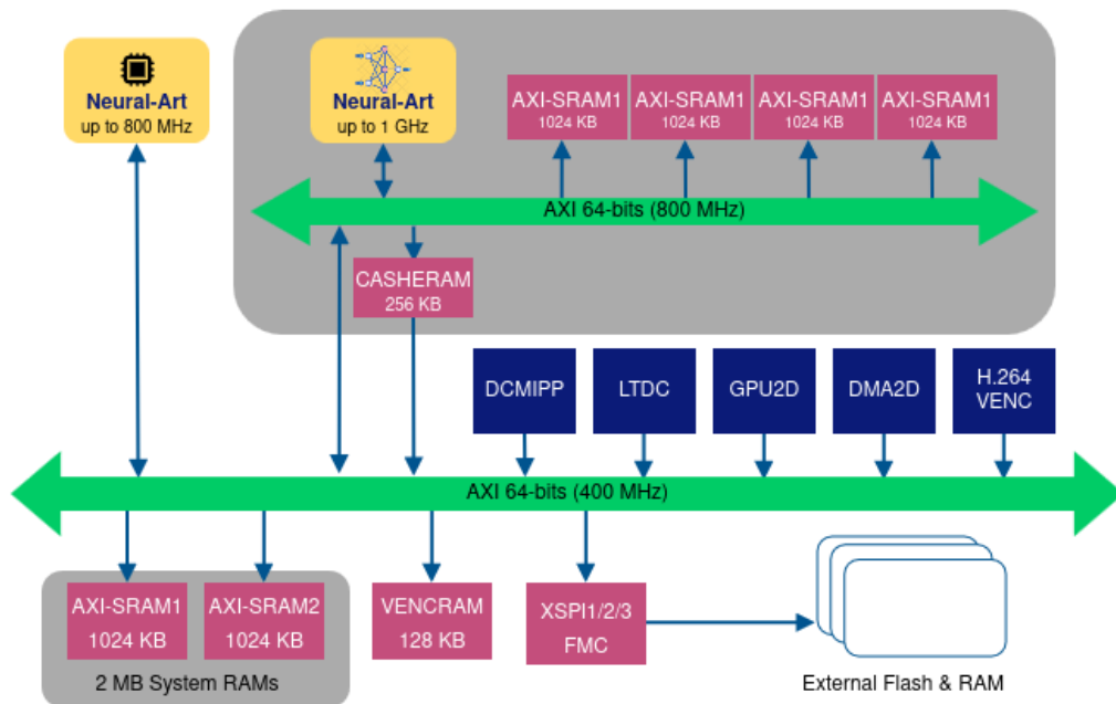
Abbildung 2.1.: STM32N6570-DK - Architektur
