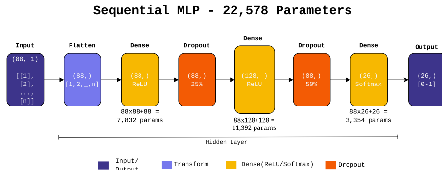
Abbildung 7.2.: Architektur des Multi-Layer Perceptrons | Eigene Darstellung
