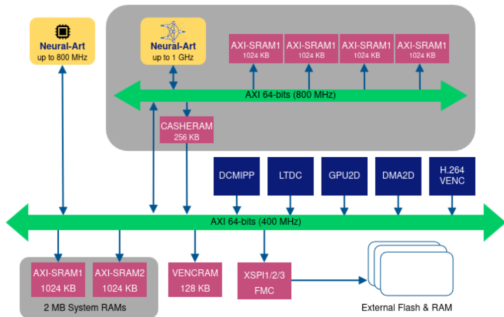
Abbildung 2.1.: STM32N6570-DK - Architektur | [10]
