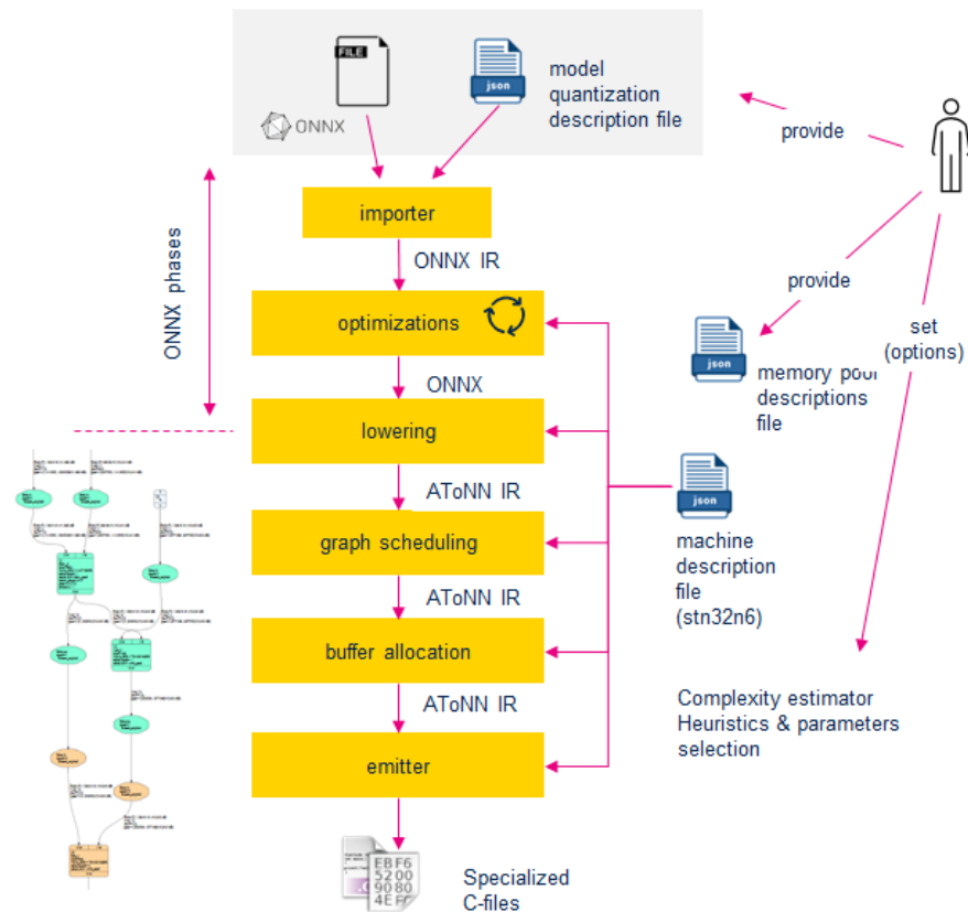
Abbildung 2.8.: NPU – Compilation ( ST Neural-ART Compiler Primer , [o. D.])
