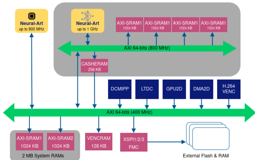
Abbildung 2.1.: STM32N6570-DK - Architektur | (STM32N6 Demo Workshop - 06 Neural Processing Unit (NPU) Theory, 2025)
