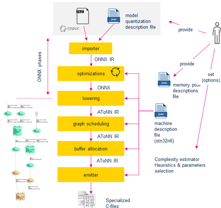
Abbildung 2.8.: NPU – Compilation [30]
