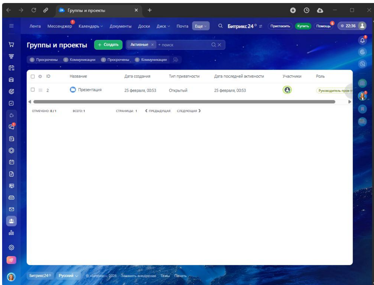
Рисунок 3.5 – Битрикс24
