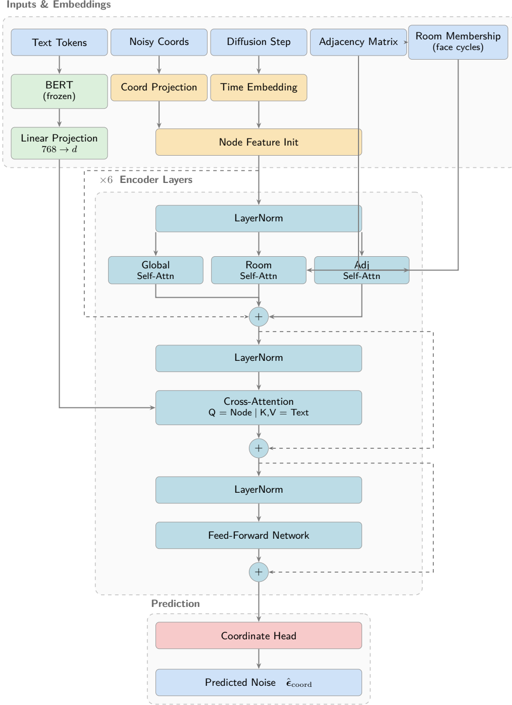
图 5: NodeDiffusionTransformer (三流) 架构图。输入的加噪坐标 \mathbf{x}_t 经坐标投影与时间步嵌入相加，构成节点初始隐向量；经 6 层三流注意力编码器处理后，节点特征经 Coordinate Head 预测坐标噪声 \hat{\epsilon}_{coord} 。
