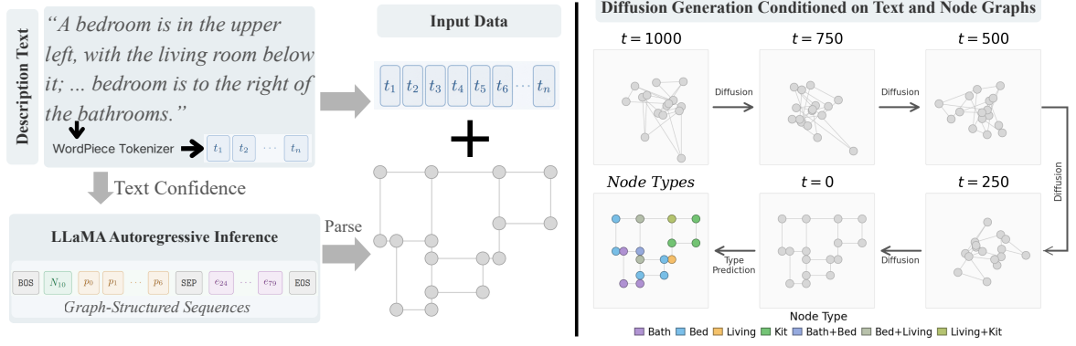
图 1: PlanDiffusion 整体流程。左: 图拓扑生成阶段以文本描述为条件, 通过 LLaMA 自回归推理生成图结构序列, 解析得到顶点图; 右: 节点坐标扩散阶段以顶点图和文本为条件, 通过 DDPM 逆扩散过程从高斯噪声 ( t = 1000 ) 逐步恢复节点坐标与类型 ( t = 0 )。
