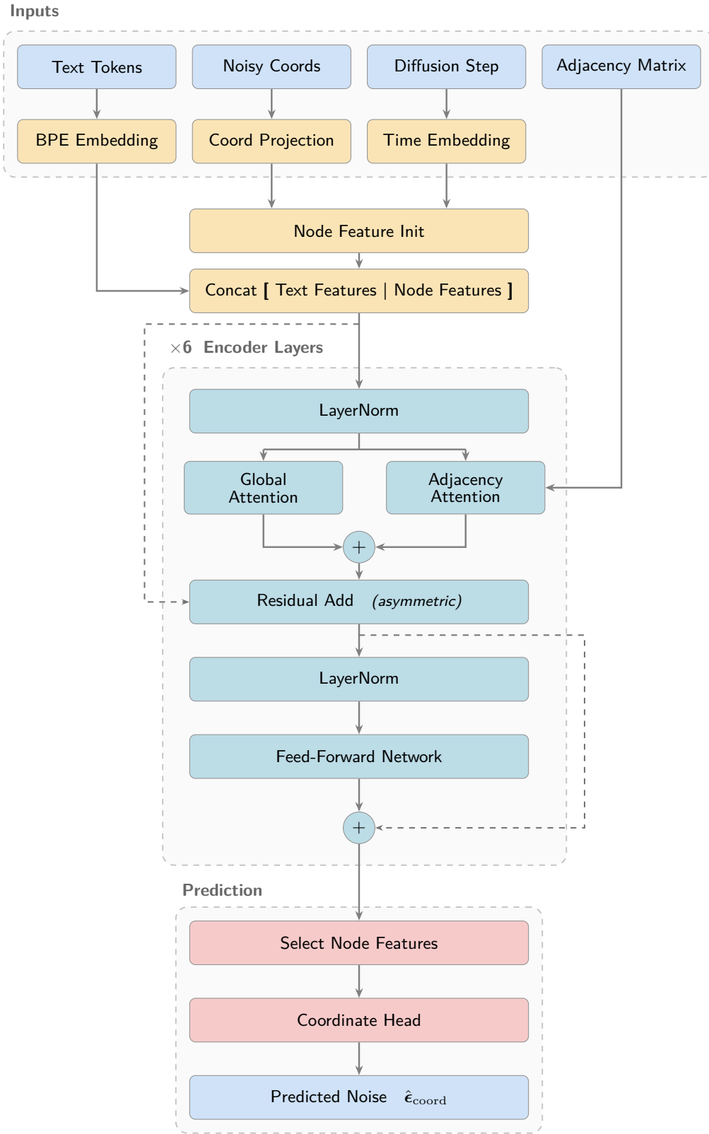
图 5: NodeDiffusionTransformer 架构图。输入的加噪坐标 \mathbf{x}_t 经坐标投影与时间步嵌入相加，构成节点初始隐向量；拼接文本嵌入后经 6 层双流注意力编码器处理；最终节点特征经 Coordinate Head 预测坐标噪声 \hat{\epsilon}_{coord} 。
