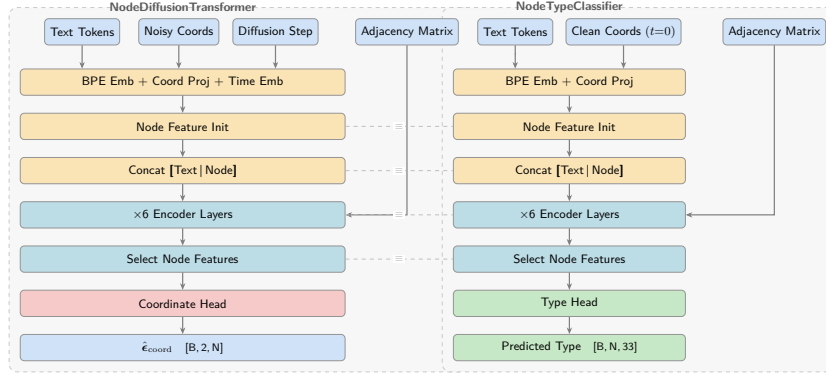
图 6: NodeDiffusionTransformer 与 NodeTypeClassifier 结构对比。两者共享同构的双流编码器设计, 但输入端 (有无时间步嵌入) 与输出头不同, 且超参数与权重完全独立。
