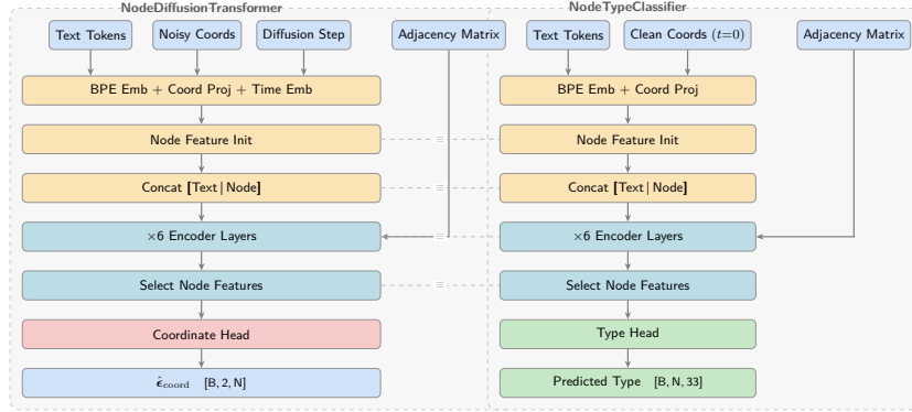
图 6: NodeDiffusionTransformer 与 NodeTypeClassifier 结构对比。两者均采用同构的双流编码器设计, 但输入端 (有无时间步嵌入) 与输出头不同, 超参数与权重完全独立。
