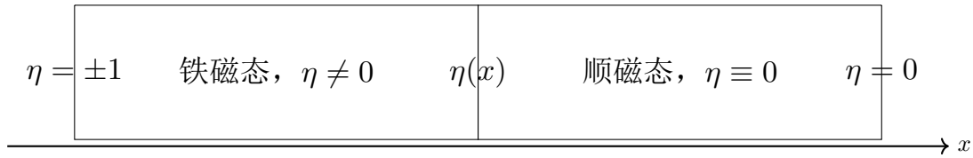
图 20: 铁磁—顺磁的局部相变
