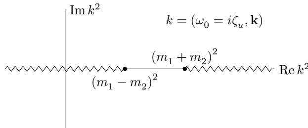
图 53: 日落图外圈积分 I(k_M^\mu) 在解析延拓下
